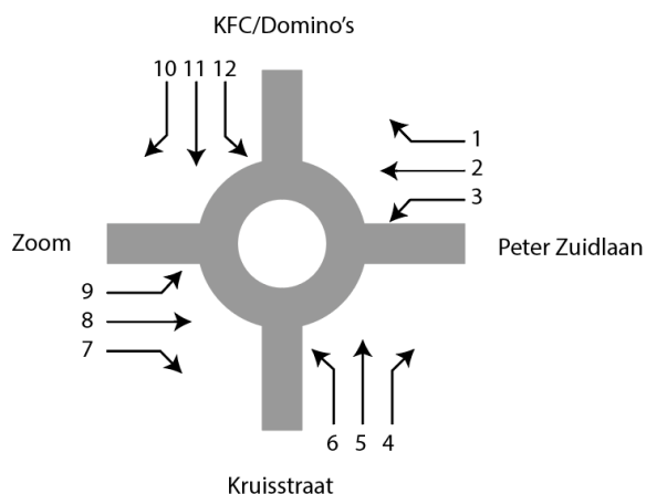
Figuur 3.3: Schema rijrichtingen
